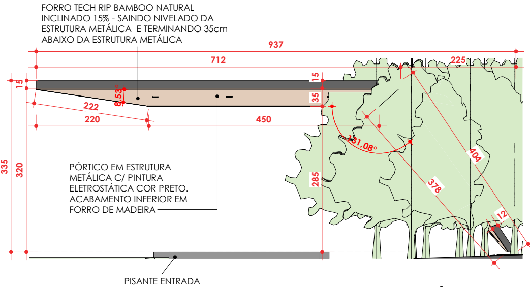
D.01 - PÓRTICO ESC:1 : 75
