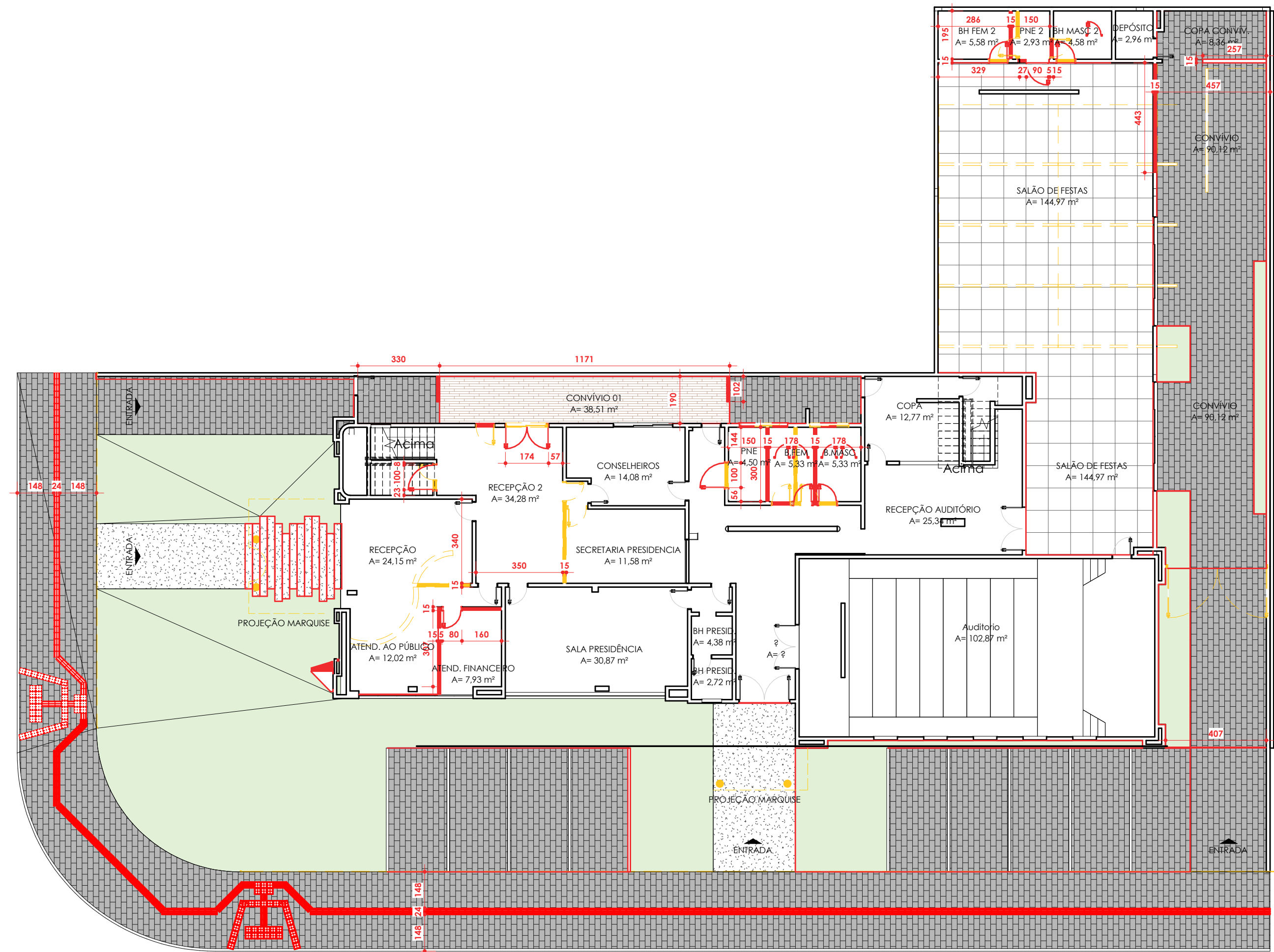
CONS./DEMOL. - TÉRREO ESC:1 : 150
