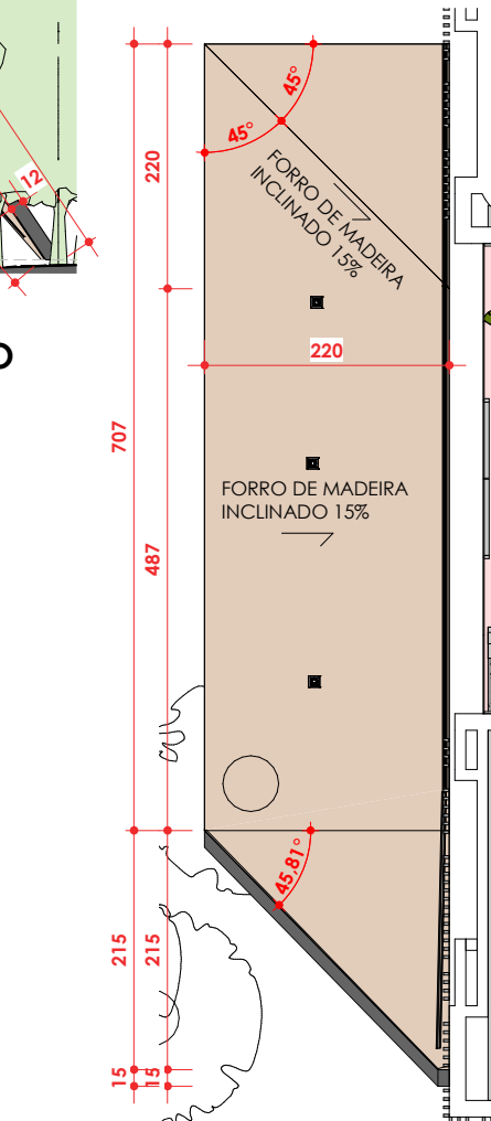
PÓRTICO - PLANTA DE FORRO ESC:1 : 75
