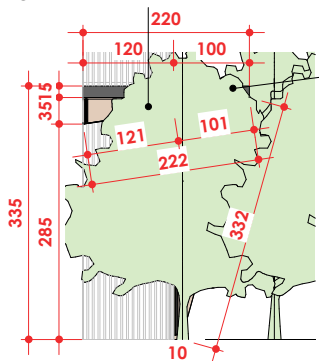
D.02 - PÓRTICO 02 ESC: 1 : 100
